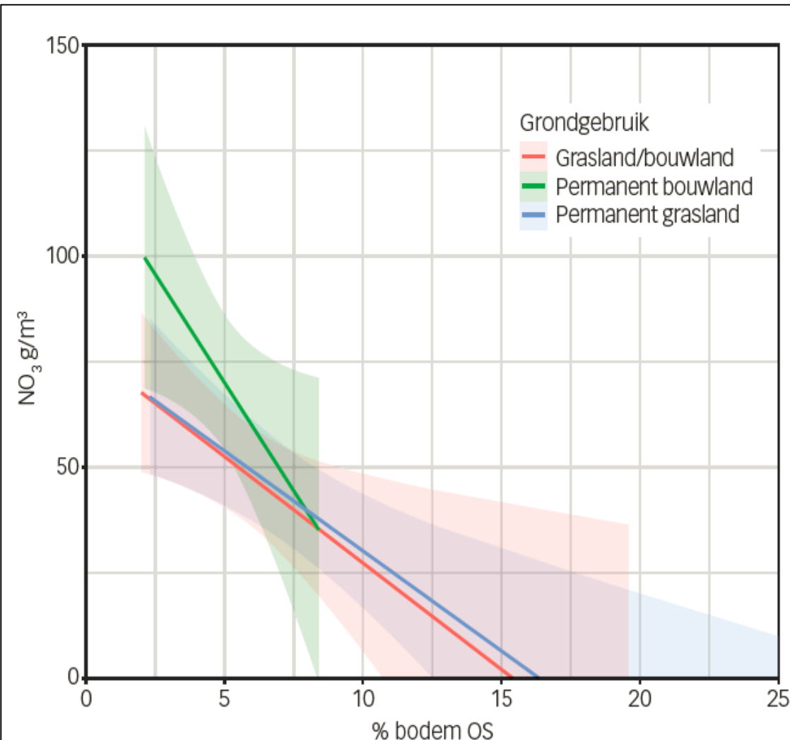
FIGUUR 2: REGRESSIELIJNEN TUSSEN NITRAATCONCENTRATIE ( \text{NO}_3 \text{ G/M}^3 ) IN HET BOVENSTE GRONDWATER EN PERCENTAGE BODEMORGANISCHE STOF (% BODEM OS) PER TYPE LANDGEBRUIK VOOR DE PERIODE 2008-2016. DE GEKLEURDE SCHADUW GEEFT HET 95 PROCENT BETROUWBAARHEIDSINTERVAL VAN DE REGRESSIELIJN AAN.
