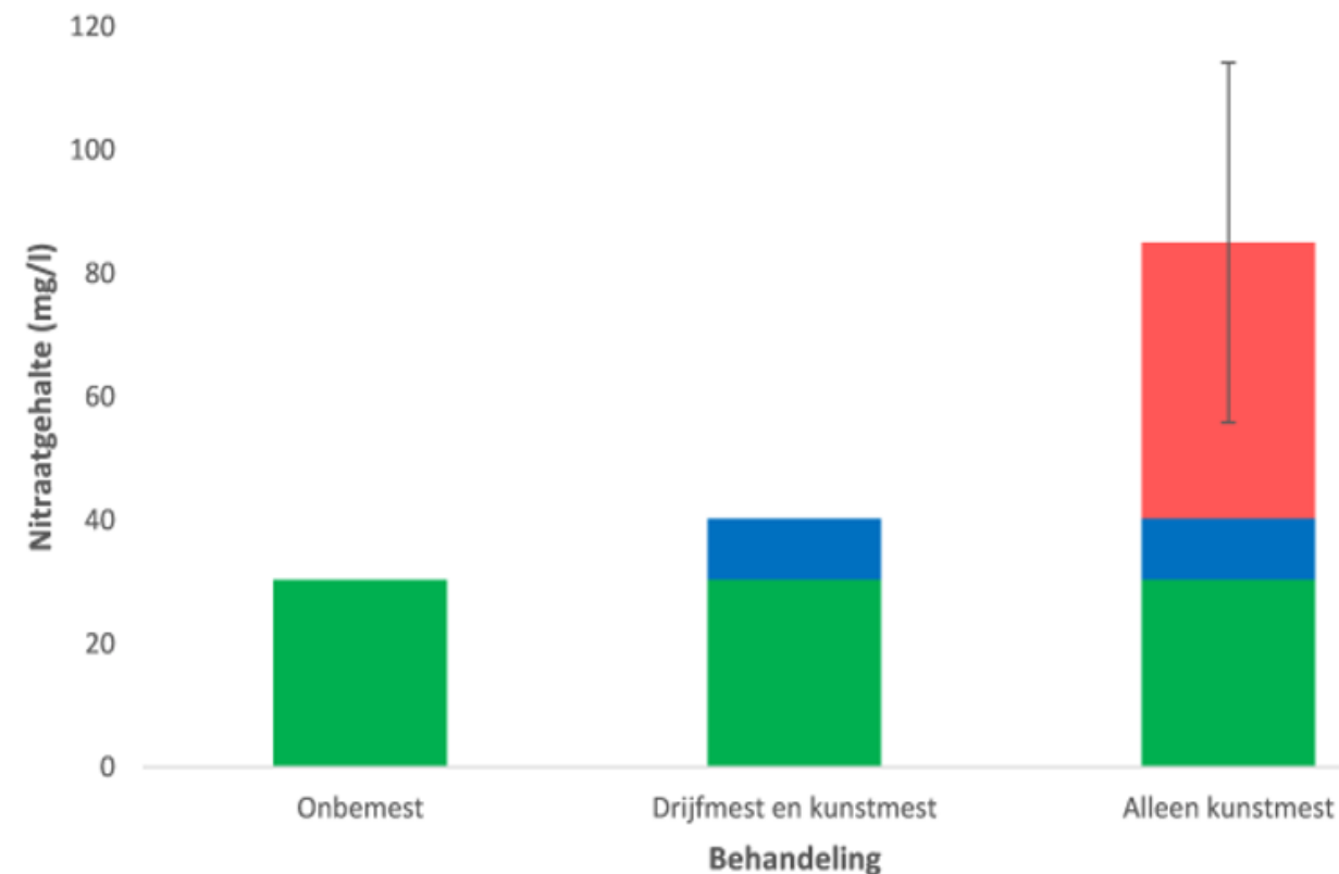
Nitraatgehalte tijdens uitspoelingsperiode in Beltrum
